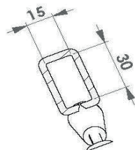
SEZ A-A
